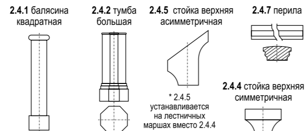
2.4.7 перила
